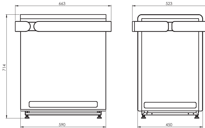
Abb.33 Abmessungen Concept R combi 9 kW und 10,5 kW
