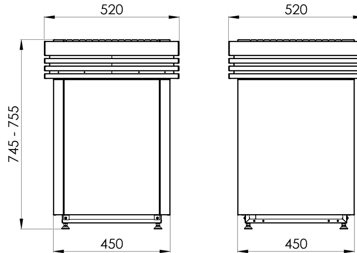
Abb.60 Abmessungen Qube 9 kW und 10,5 kW (QUBE-090 / QUBE-105) Maße in mm
