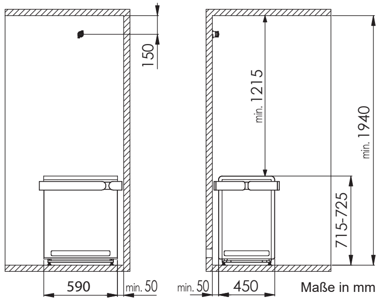
Abb.32 Sicherheitsabstände Concept R combi 9 kW und 10,5 kW (CP-RCB-090 / CP-RCB-105)
