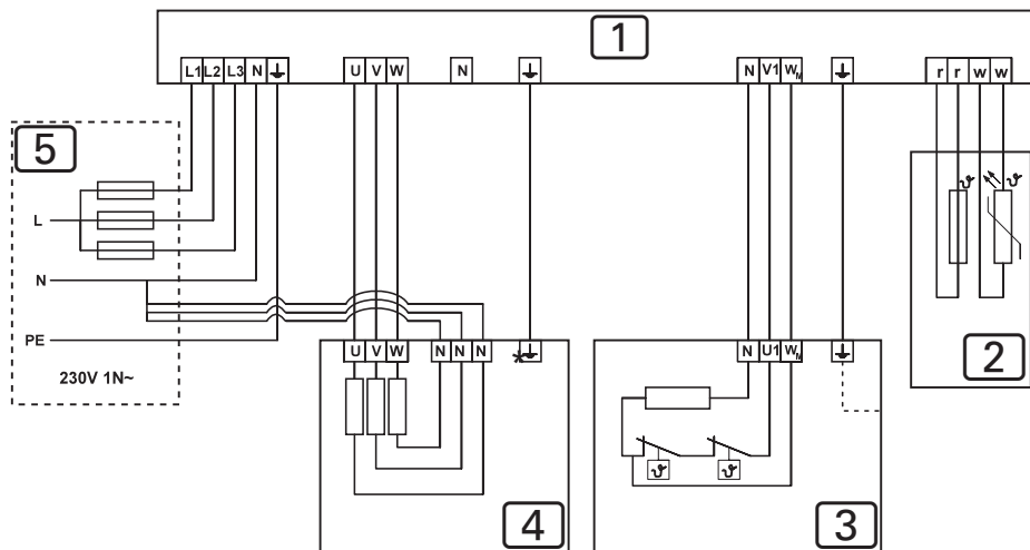
Bild 6 Kopplingsschema 230 V 1 N~ Home combi 6,0 kW och 9,0 kW (HOME-C60/HOME-C90)
