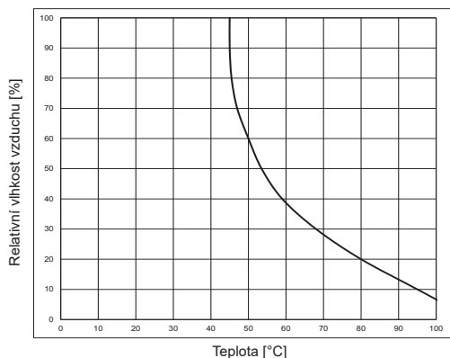
Obr. 7 Charakteristika teploty / relativní vlhkost vzduchu (odpovídá normě EN 60335-2-53)
