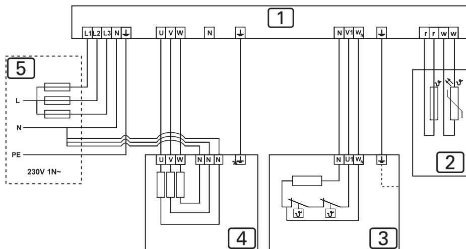
Kuva 6 Liitäntäkaavio, malli 230 V 1N~ Home combi 6,0 kW ja 9,0 kW (HOME-C60 / HOME-C90)
