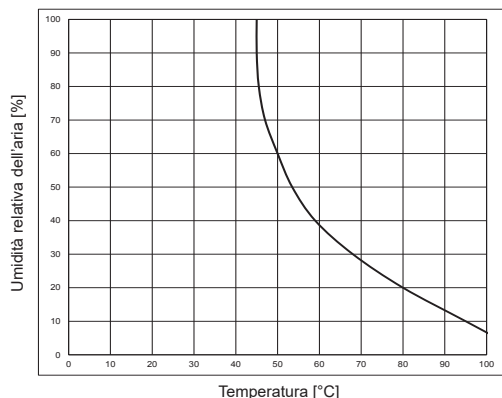
Fig. 7 Curva caratteristica temperatura / Umidità relativa dell'aria (conforme a EN 60335-2-53)
