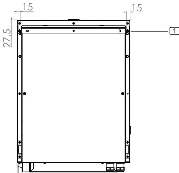
afb. 3 Positie van de montagelijst Home combi Afmetingen in mm
